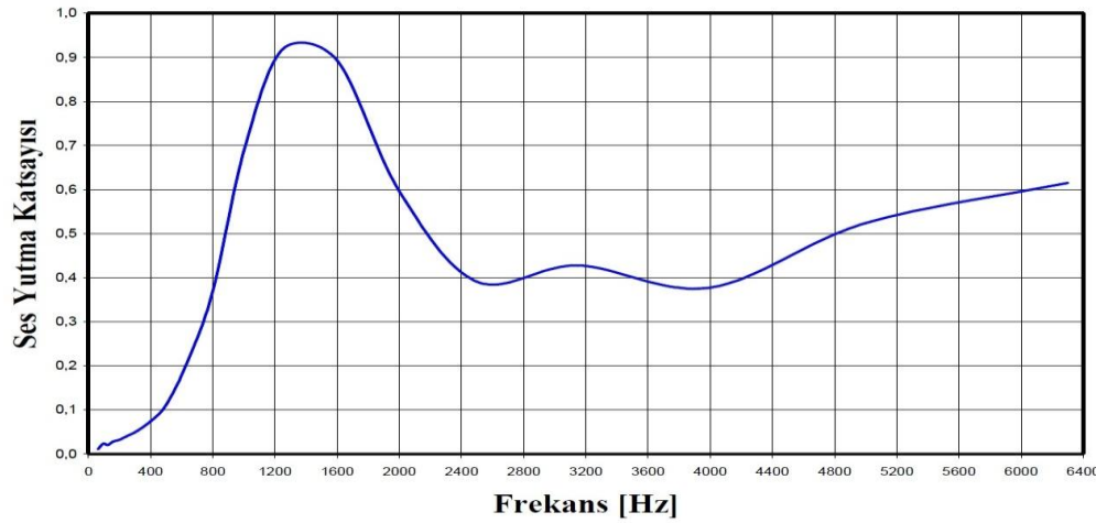
Şekil 4. "Polietilen sünger (kalınlık: 30 mm)" malzemesinin ses yutma katsayısının frekansa bağlı olarak değişimi.
